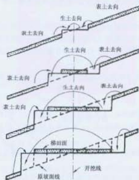
图7 表土逐行置换法
